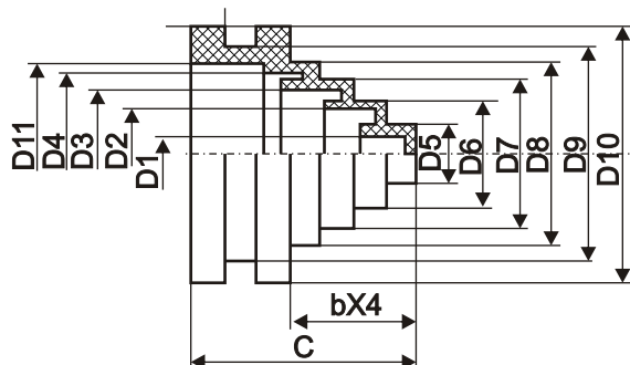
Рис. 14.1.1 Ввод сальниковый
